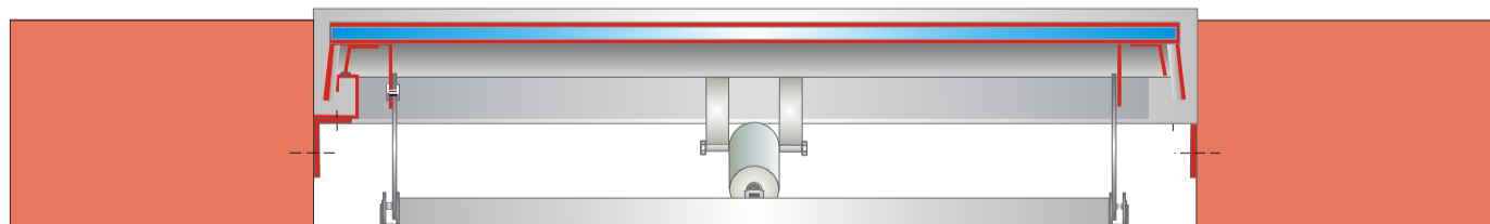
Coupe horizontale
